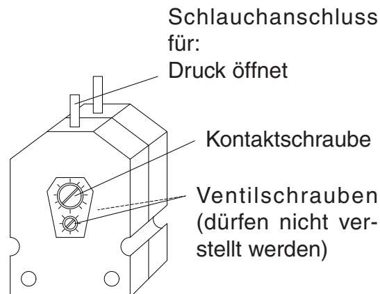
Druckwellenschalter
