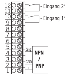
Klemmleiste X4 (für Lichtschränke 3-Draht PNP oder NPN)
